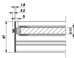
Met Borstel dichting avec joint brosse
