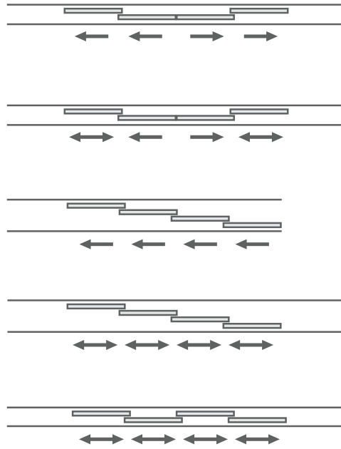
Met een rails verlenging Avec prolongement du rail
